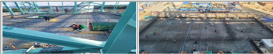
[사진] 실족방지용 근로자 작업통로 미설치 현장사진
